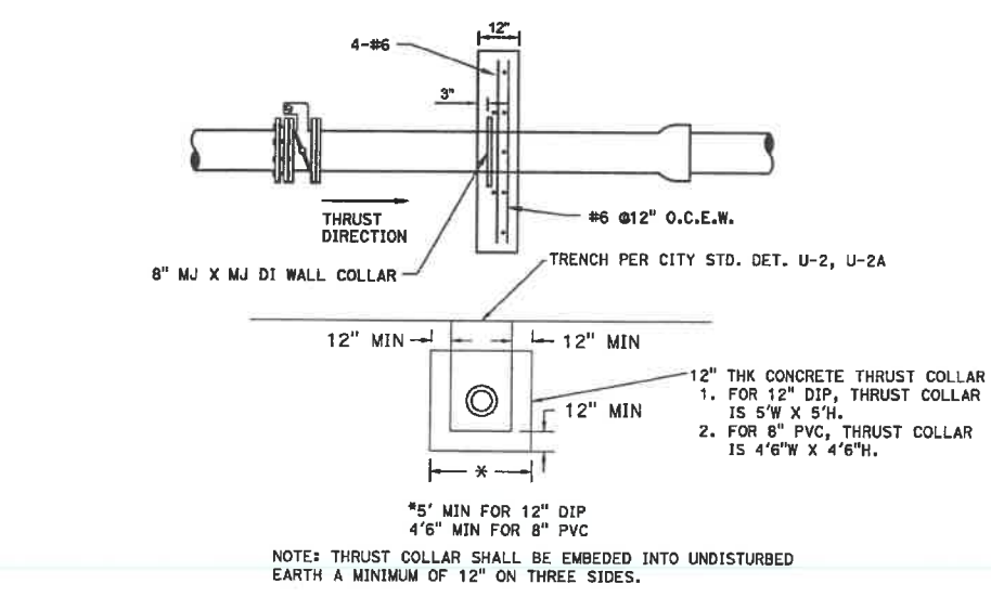
5 THRUST COLLAR Scale: 1" = 5'
